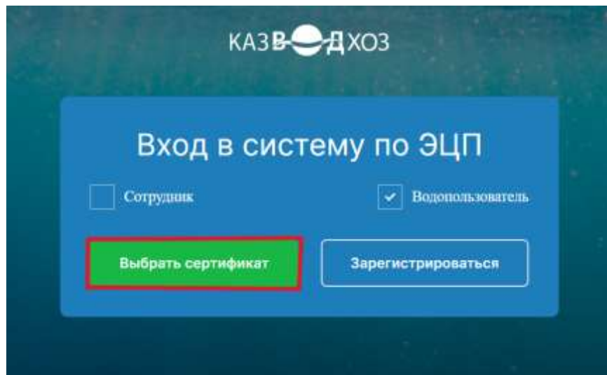
Рисунок 3. Начало авторизации
