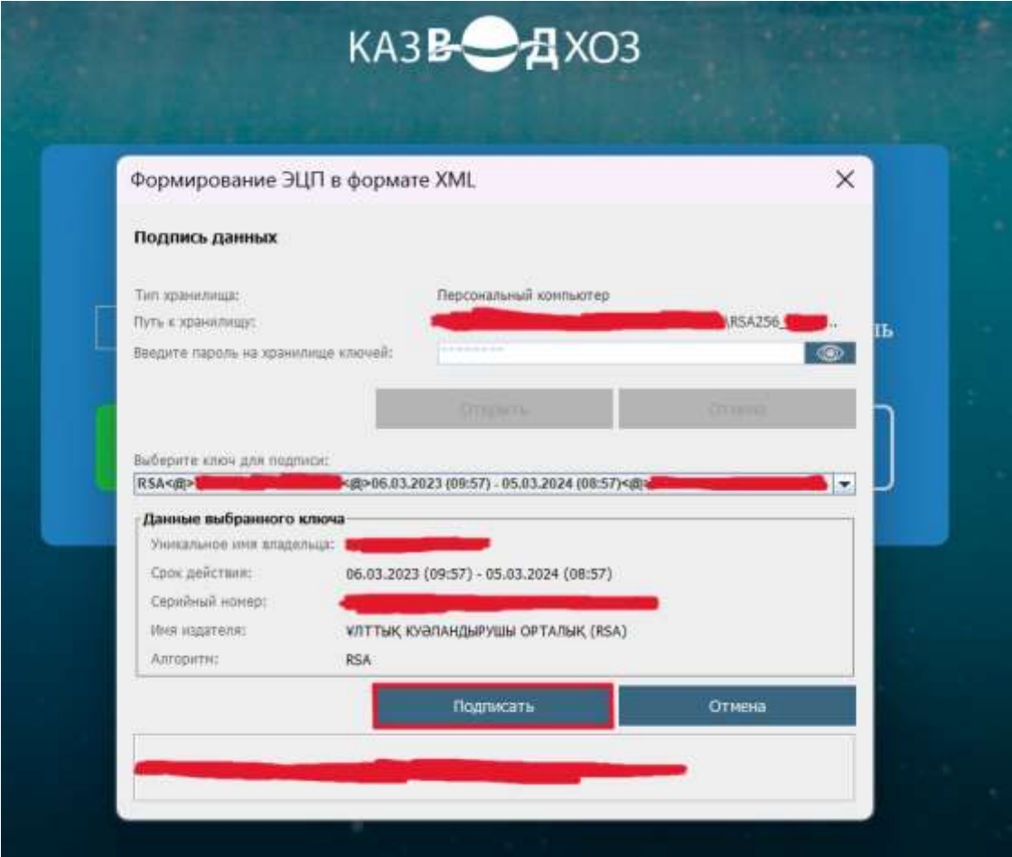
Рисунок 7. Окно подписи
